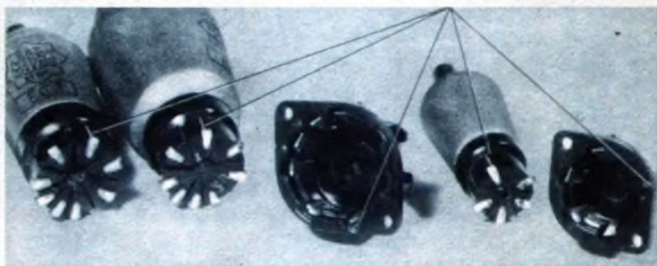
Nur wenn Marke auf Marke kommt, läßt sich die Röhre in die Fassung ein-schieben. (Werkphoto Telefunken)
