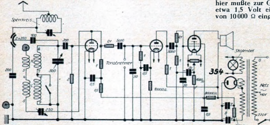
HF- und NF-mäßig unterscheidet sich diese Schaltung nicht von der des »München«, wohl aber ist die Stromversorgung aus dem Netz eine andere.
