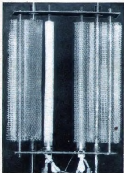
Die beiden elektrisch getrennten Gleichrichterstreifen der CY 2. Der Anodenmantel des linken Systems ist zurückgebogen, um zu zeigen, wie eng Kathode und Anode beieinanderstehen. (Phot. Herrnkind)
