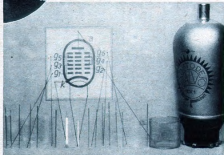
Alle Teile, die im Vordergrund aufgerichtet stehen, befinden sich mit größter Präzision ineinandergeschieben innerhalb der Röhre. (Werkphoto Valvo)
