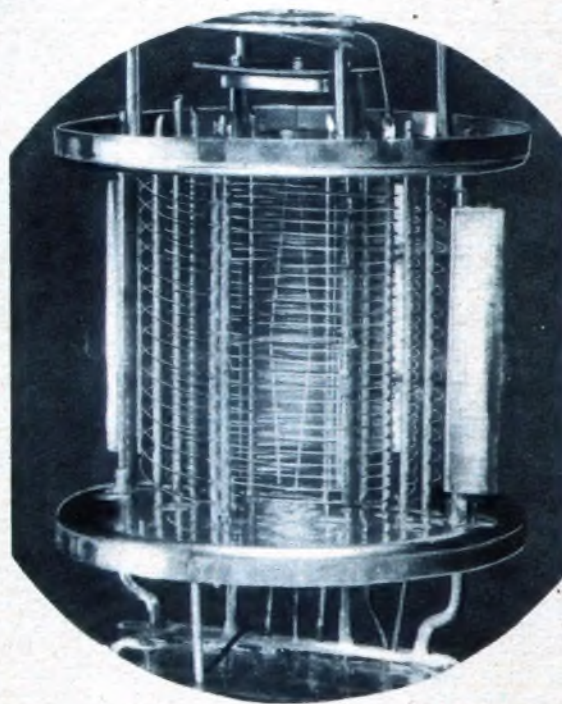
Durch dieses Gewirr von Drähten müssen die von der Kathode ausgehenden Elektronen hindurch, um so das zu vollbringen, was wir von Röhren verlangen. Wir sehen hier die Achtpol-Röhre KK 2 teilweise aufgeschnitten. (Phot. Herrnkind)
