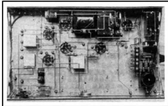
Links ein Blick unters Paneel und rechts die Draufsicht.
