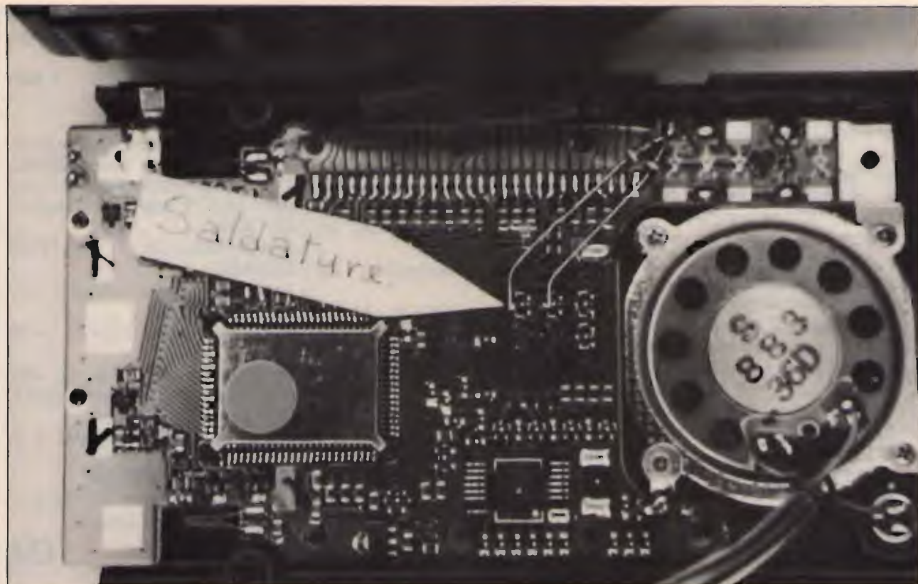
figura 5 Individuazione dei punti di saldatura dei catodi.
