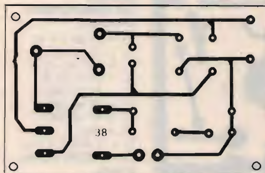
figura 2 Circuito stampato del dispositivo di protezione per diffusori acustici, in scala 1:1.
