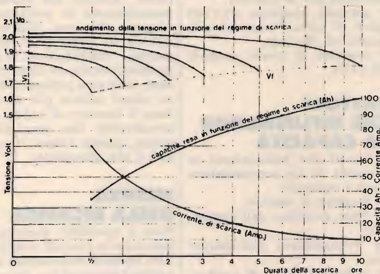
Curve di scarica ai regimi di 10-5-3-2-1-1/2 ore di elementi serie "SM" (valori riferiti a C10 = 100 Ah) - Temperatura 25 °C - Densità elet. 1,25g/cm³
