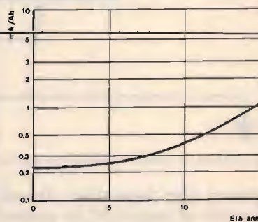
figura 16 Andamento della corrente di mantenimento in funzione dell'età della batteria, alla tensione di 2,23 \pm 1\% V/elemento.
