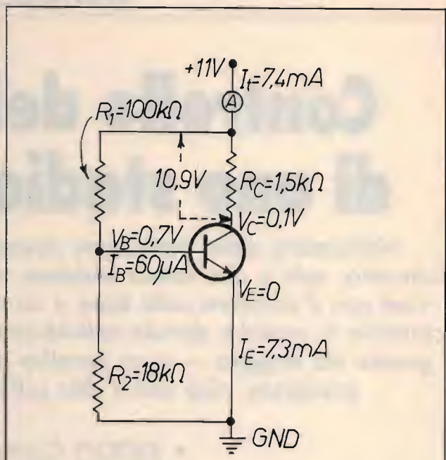
figura 2 Il cortocircuito del condensatore elettrolitico collega direttamente a massa l'emettitore. Aumenta così di molto la IB, e, conseguentemente, il transistor va in saturazione. Aumenta anche la IC, che però è limitata da RC. Notare il valore della VCE di saturazione (0,1 V).
