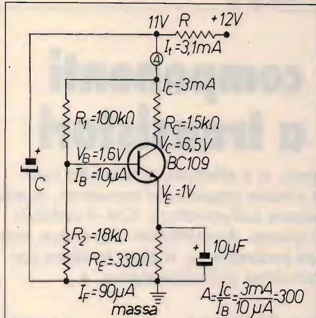
figura 1 Schema classico di uno stadio audio a transistore, in classe A, con configurazione a emettitore comune: il segnale entra sulla base ed esce dal collettore. È stabilizzato con partitore sulla base e resistore d'emettitore. Il resistore R e l'elettrolitico C costituiscono la rete di disaccoppiamento. L'amperometro misura la corrente di collettore del transistore (3 mA) e la piccola corrente nel partitore (circa 0,1 mA).
