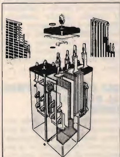
figura 4 Sezione di un accumulatore utilizzando piastre positive tubolari.
