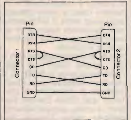
figura 3 Schema dell'eliminatore di modem RS-232.
