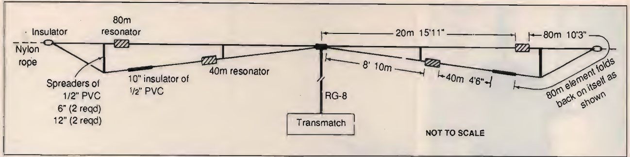
figura 2 "Schema del dipolo (non in scala), della lunghezza compresa tra 12,2 e 12,5 metri; risona su 10, 20, 40 e 80 metri e, con un adattatore, funziona bene su ogni banda HF". Nylon rope: tirante di nylon; Resonator: trappola; Spreaders: distanziatori; 80 m elements fold back...: l'elemento per gli 80 metri è ripiegato su sé stesso come mostrato in figura.
