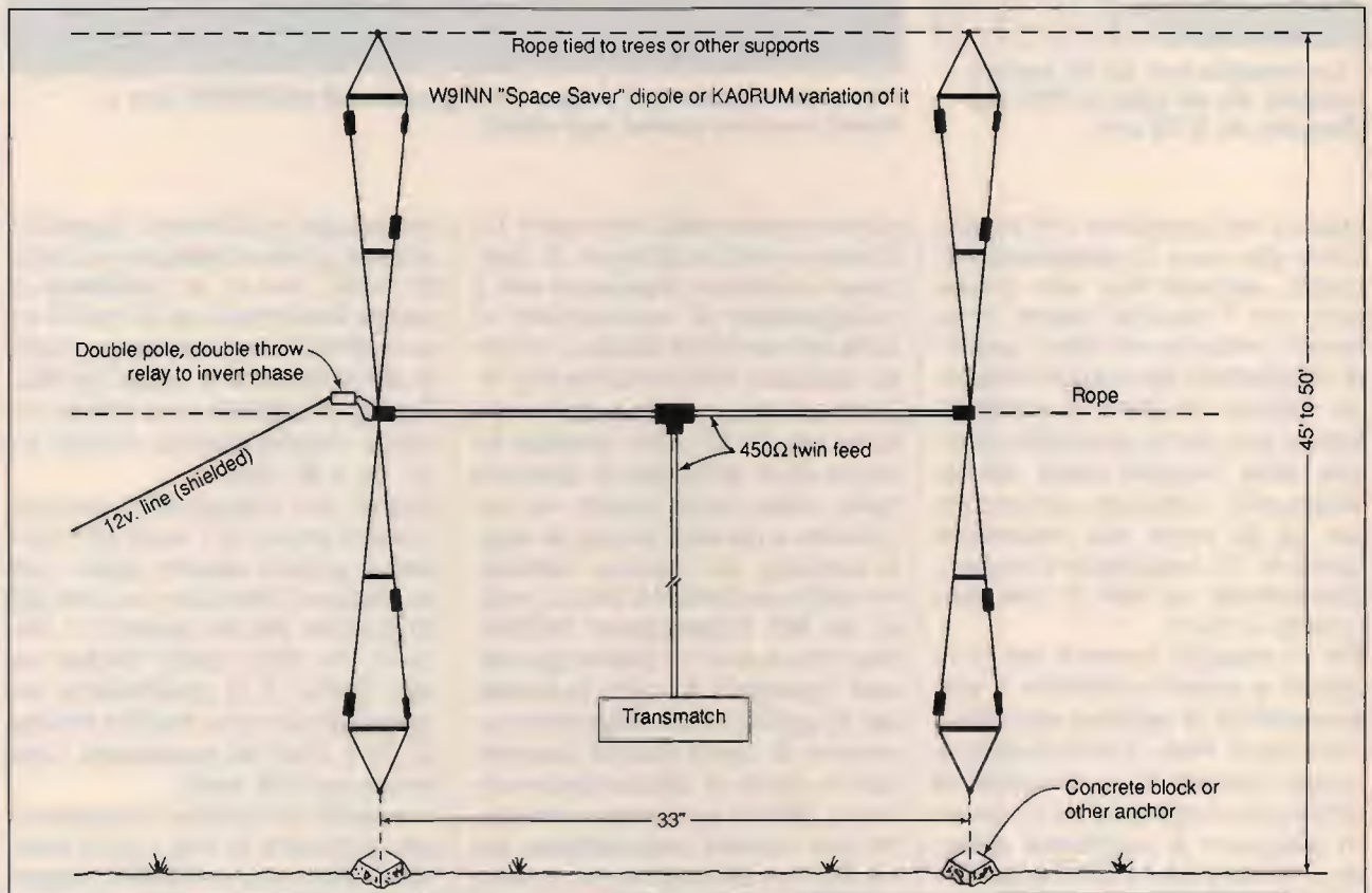
figura 3 "La differenza di fase del sistema può essere selezionata tra 0° e 180° per modificare l'irradiazione. Il guadagno è compreso tra 0,2 e 4,9 dB rispetto al dipolo singolo. Lobi multipli si verificano sulle frequenze più alte". Rope tied...: tirante appeso agli alberi o altri supporti; Double pole...: relè per inversione di fase; 450 ohm twin feed: piattina bifilare da 450 ohm; Concrete block...: blocco di cemento o altro ancoraggio; 12 V line (shielded): alimentazione schermata per 12 V; 45' to 50': 13,7-15,24 metri; 33': 10 metri.
