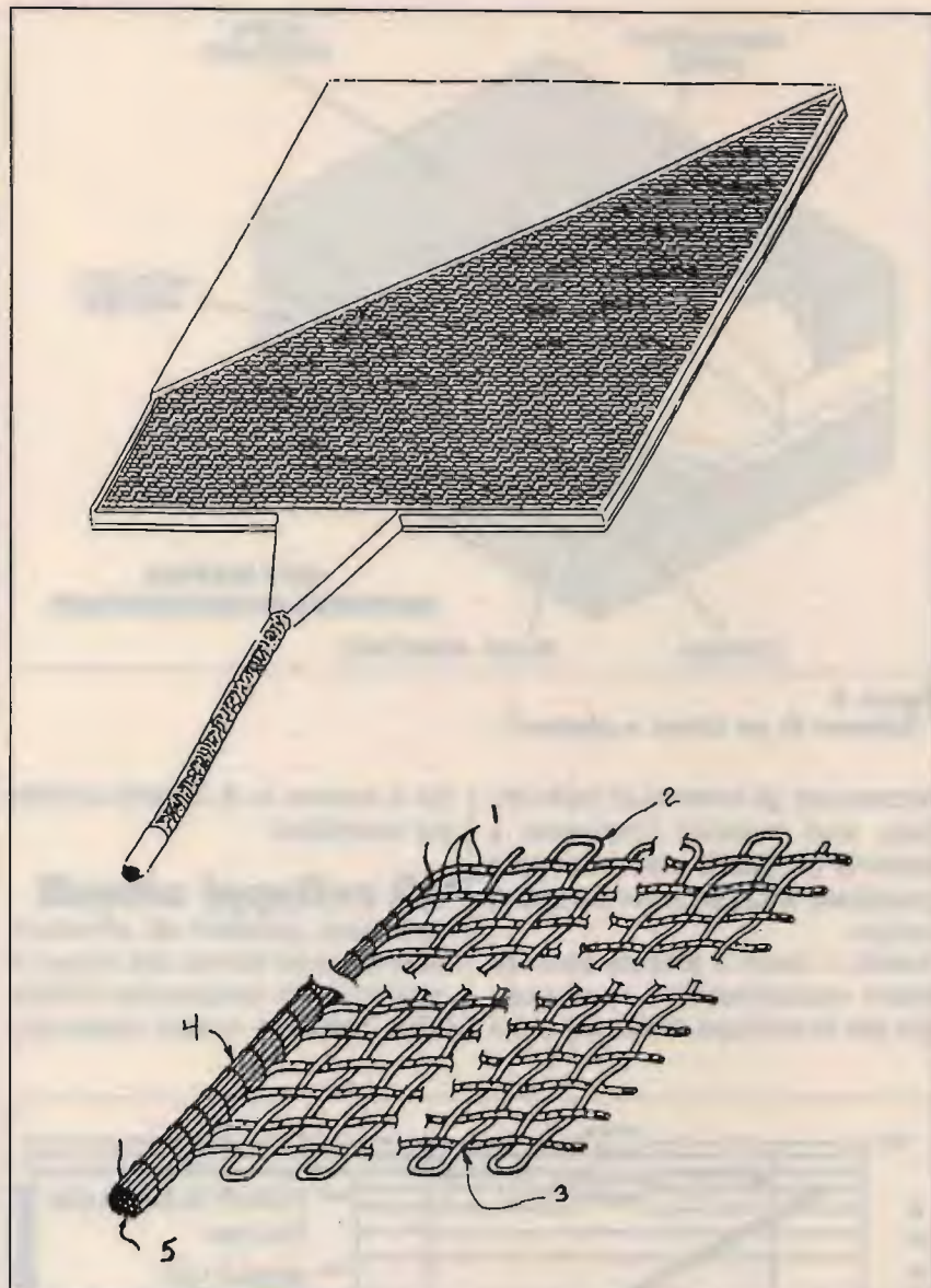
figura 8 "Un sistema a fibre ottiche per la produzione dell'illuminazione di fondo in un visore a cristalli liquidi, per renderlo leggibile anche in condizioni di scarsa luce ambientale. Le fibre ottiche (1) vengono tessute con una trama convenzionale (2) per creare un'ondulazione delle strutture ottiche (3). Le estremità vengono riunite in un cavo (4) che viene poi tagliato e lucidato (5)".
