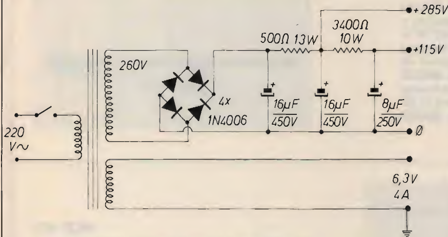
Schema di alimentatore da rete per ricevitore inglese Redifon R-50 M.
