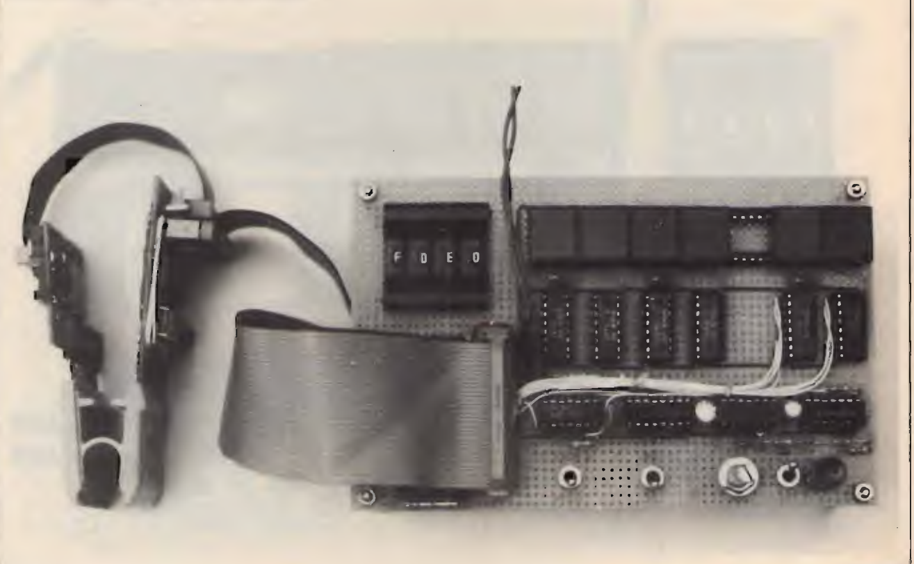
foto 7 Vista d'insieme con tutti i cavi collegati.
