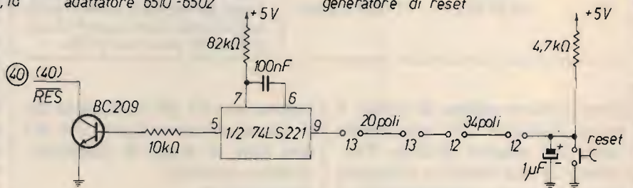
adattatore 6510 - 6502
