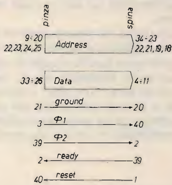
adattatore 6502 - 6510
