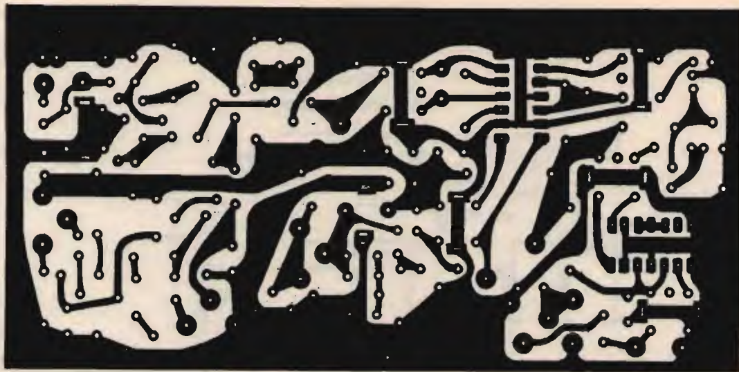
CIRCUITO STAMPATO
