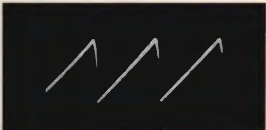
foto 7 Forma d'onda rilevata ai capi del trimmer P_2 .
