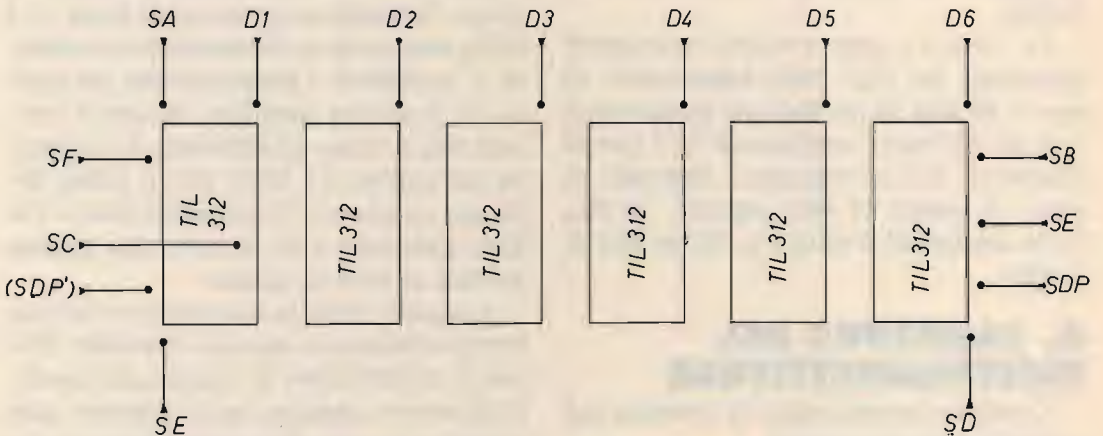
figura 19 Disposizione dei componenti del display.
