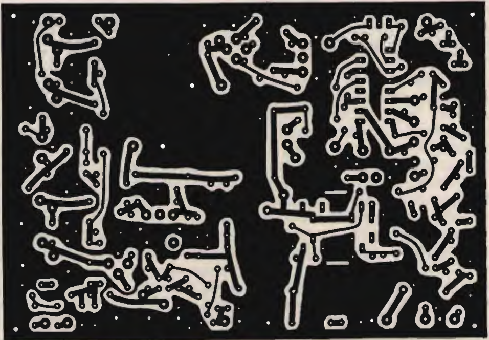
figura 12 Circuito stampato del modulo RX.
