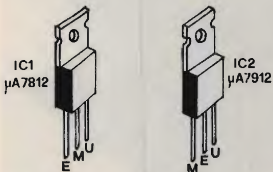
figura 8 Disposizione componenti.
