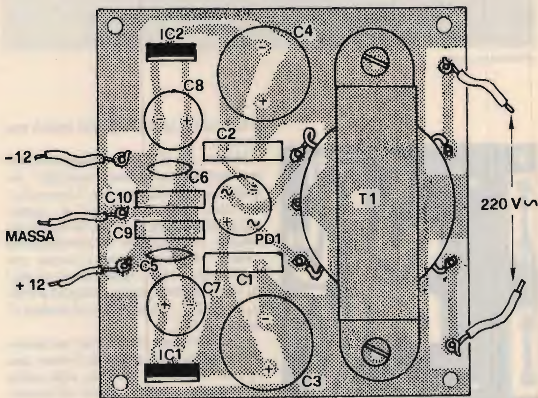
figura 8 Disposizione componenti.
