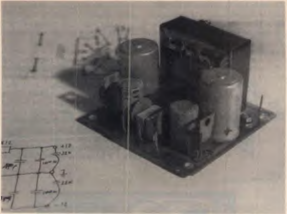
Alimentatore duale.
