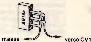
Sostituzione del BA102 con un BB135.
