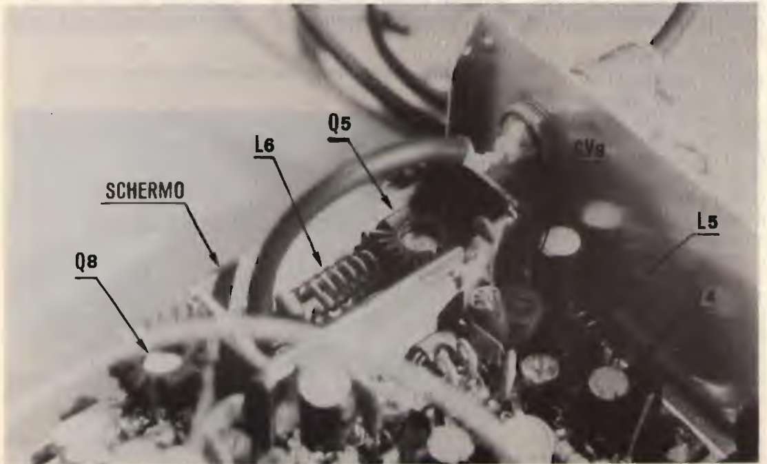
Vista (parziale) dello stadio finale RF e della schematura dello stesso in un prototipo del "Gamma Leonis".
