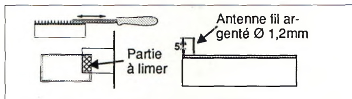
Figure 9. Limer les traversées pour qu'elles affleurent presque.
