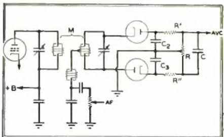
FIG. 65E. PHASE-SHIFT DISCRIMINATOR
