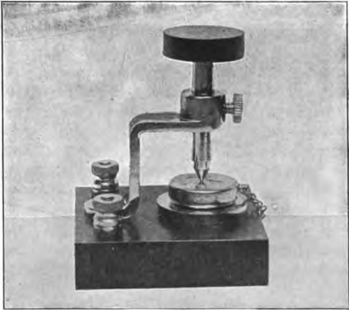
FIG. 16.—SILICON DETECTOR.
