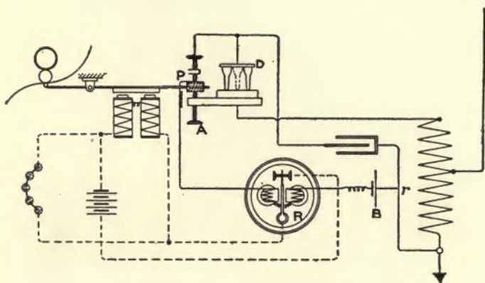
FIG. 211.—BRANLY-POPP RECEPTOR.
