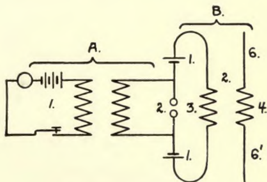
FIG. 176.—BRAUN TRANSMITTER.
