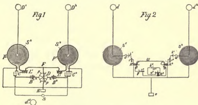
FIG. 301.—TESLA DUPLEX SYSTEM.
