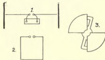
FIG. 289.—BJERKNÆS RESONANCE APPARATUS
