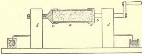
FIG. 132.—CALZECCHI TUBE.
