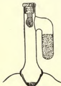
FIG. 147.— DUCRETET COHERER.
