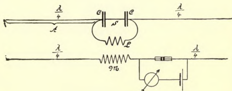
FIG. 197.—BRAUN RESONATOR.
