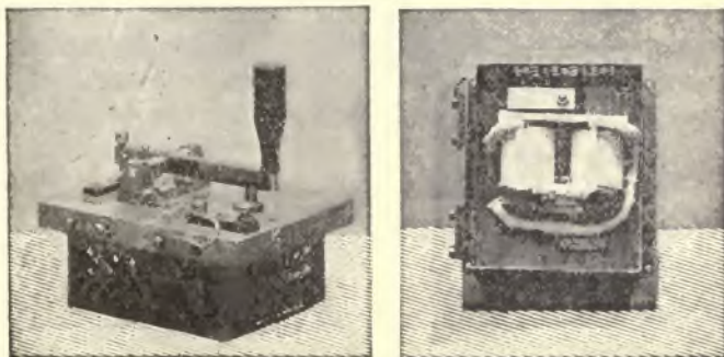
FIG. 220a,b.—BRAUN KEY.
