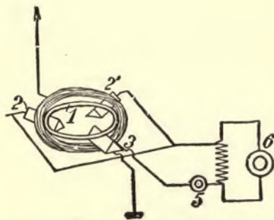
FIG. 151.— HERTZIAN DETECTOR. (Second Form.)
