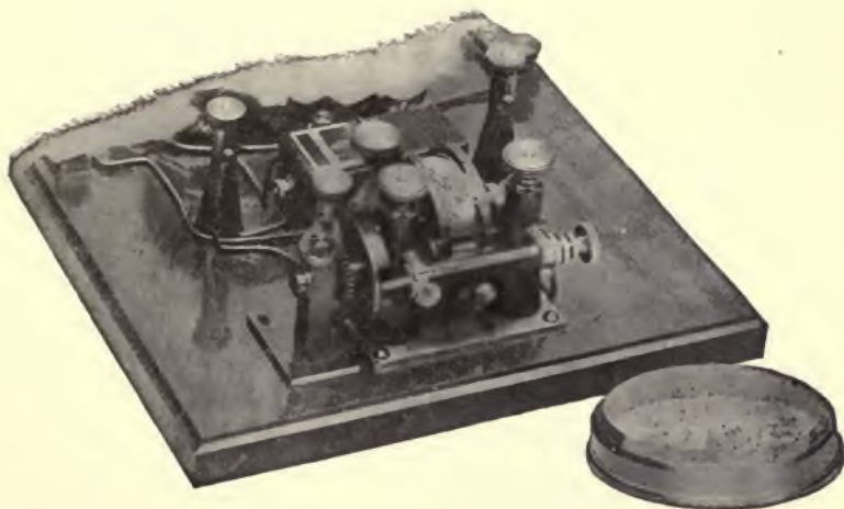
FIG. 236.—BRAUN DE-COHERER.
