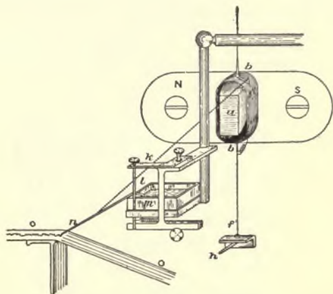
FIG. 246.—SIPHON RECORDER.
