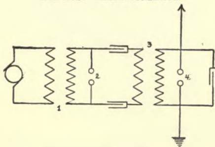
FIG. 127C.—TESLA OSCILLATOR.
