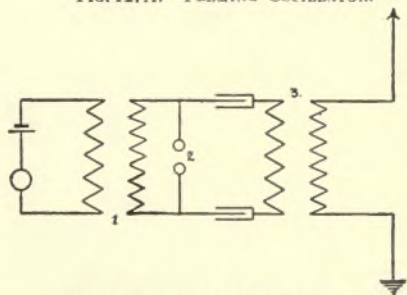
FIG. 127B.—BRAUN OSCILLATOR.
