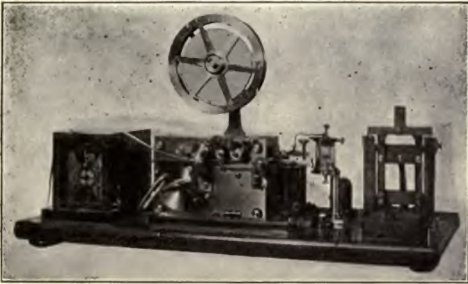
FIG. 212.—BRANLY-POPP RECEPTOR.
