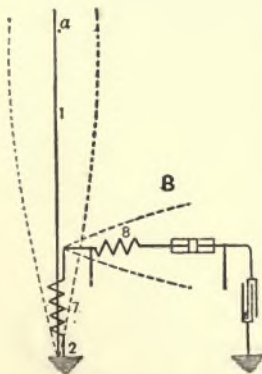
FIG. 195.—SLABY-ARCO RECEPTOR.
