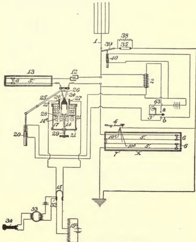
FIG. 204.—FESSENDEN SYSTEM.
