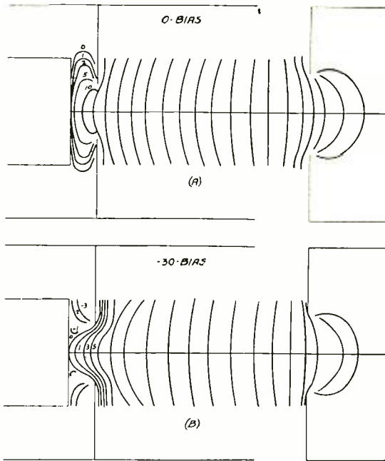
Fig. 8—Equipotential surfaces in proximity of cathode.
