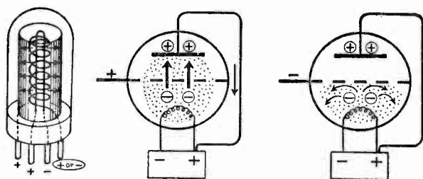
DE FOREST AUDION OR TRIODE
