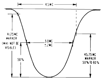
Fig. 3 IF CURVE
