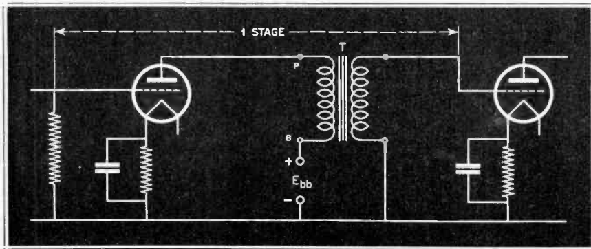
Fig. 1. Transformer-coupled triodes.
