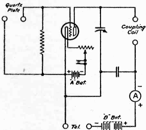
Fig. 1. Piezo Oscillator Circuit.
