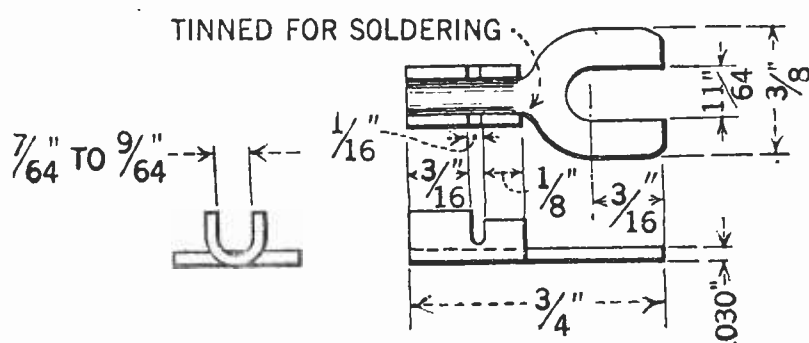
FIG. 3 The standard lug
