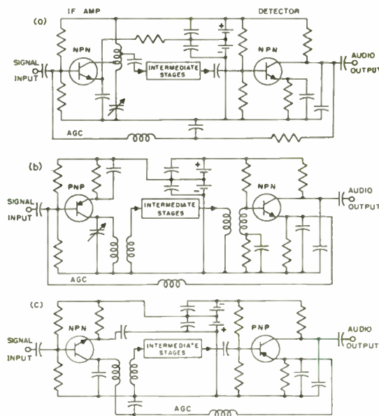
Fig. 19—AGC circuits.
