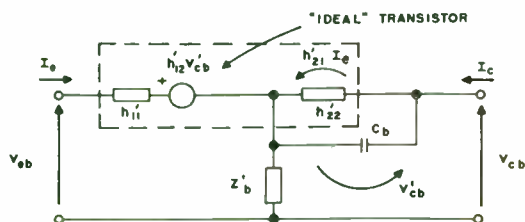
Fig. 2—"Real" transistor.
