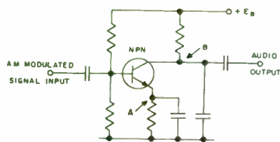
Fig. 16—Transistor detector circuit.
