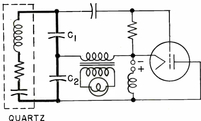
Fig. 5—Hansen.
