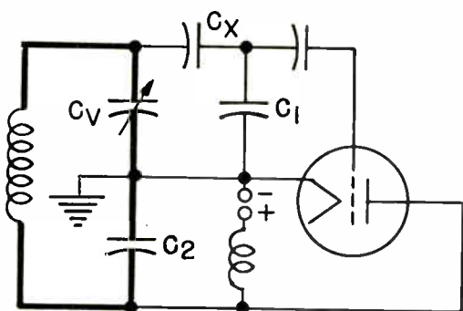
Fig. 3—Vackar.
