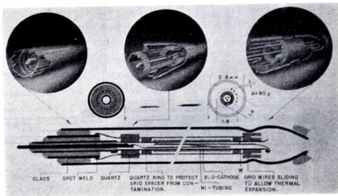
Fig. 14—Subminiature triode.
