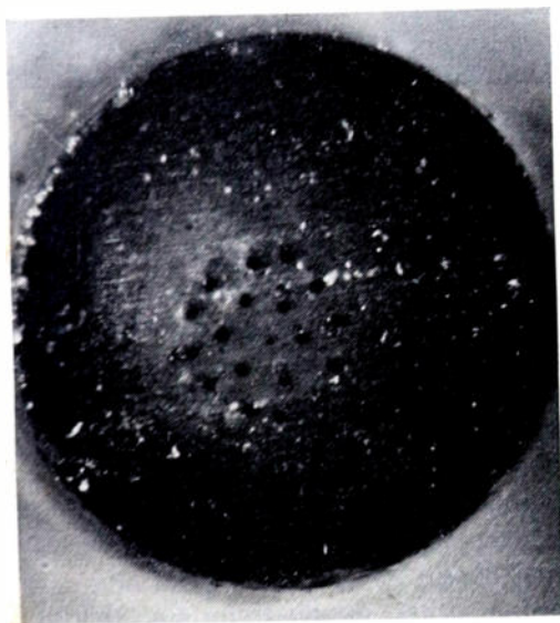
Fig. 12—19-electrode configuration, top view ( 12\mu wires).
