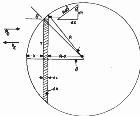
Fig. 16—Rough-moon reflection
