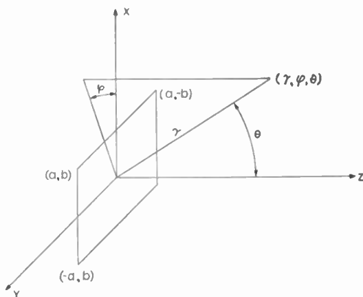
Fig. 2—Rectangular antenna.
