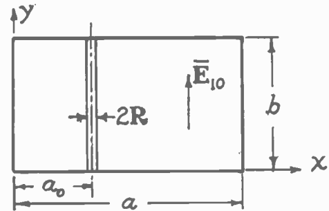
Fig. 5—Transverse wire.
