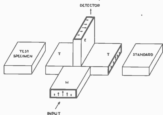
Fig. 6—Magic Tee.
