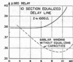
Fig. 21B—Delay.
