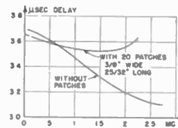
Fig. 23B—Delay.
