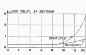
Fig. 25B—Delay.
