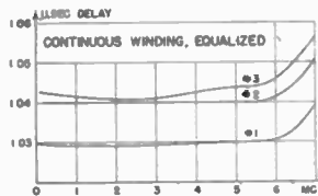
Fig. 20B—Delay.
