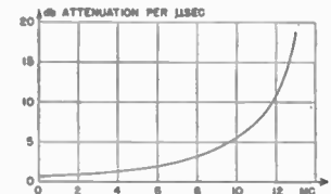
Fig. 25C—Attenuation.
