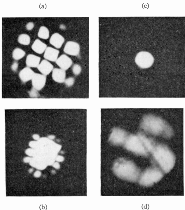
Fig. 1—(a) VA_2 = 800 (b) VA_2 = 885 (c) VA_2 = 960 (d) VA_2 = 1170 .
