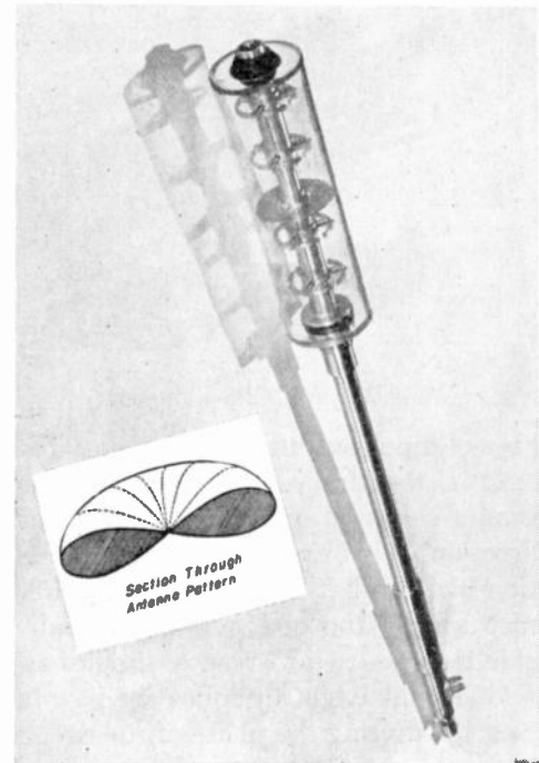
Fig. 55—“Bups” antenna.
