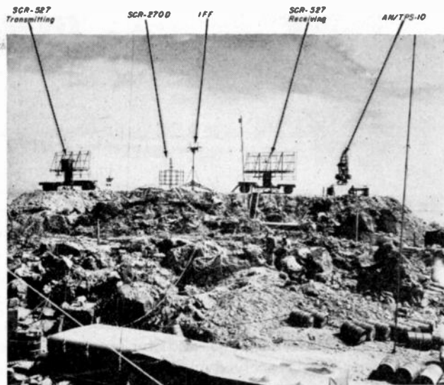
Fig. 80—Radar on Iwo Jima.
