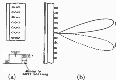
Fig. 58—"Eagle" antenna.
