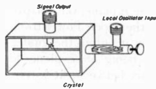
Fig. 45—Wave-guide mixer.
