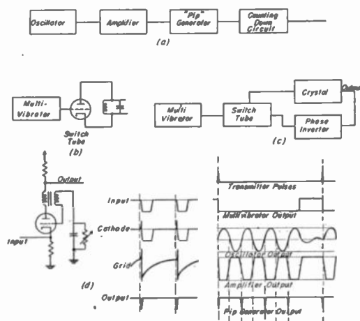
Fig. 71—Range-mark circuit.
