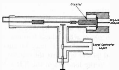
Fig. 44—Crystal mixer.
