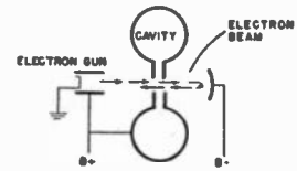
Fig. 21—Reflex klystron.
