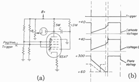
Fig. 69—Phantastron.
