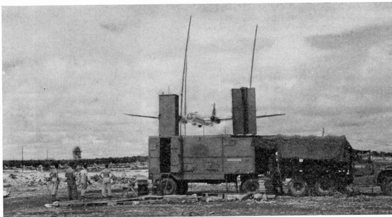
Fig. 86—AN/MPN-1 on Guam.
