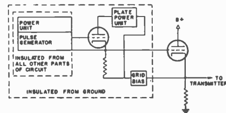
Fig. 14—Hard-tube modulator.
