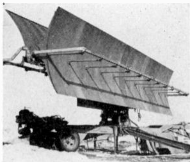
Fig. 57—AN/CPS-1 antenna.
