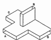
Fig. 41—"Magic T."
