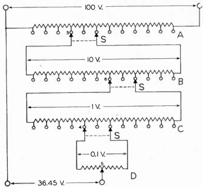
Fig. 5—100,000-ohm Thomson-Varley potentiometer.
