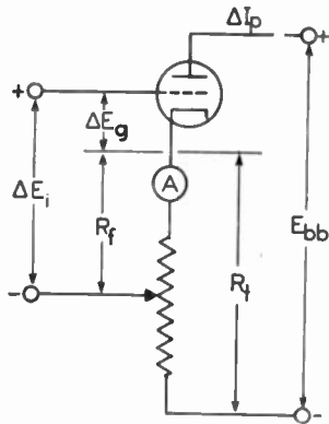
Fig. 2—Basic circuit.
