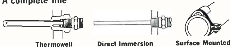
Thermowell
