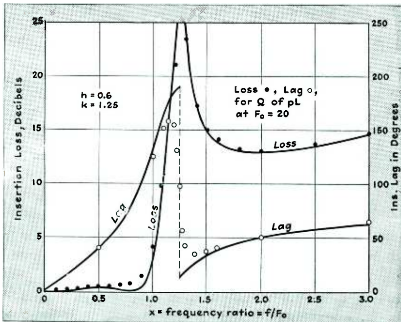
Fig. 5—More detailed data for parameter values h=0.6 , k=1.25
