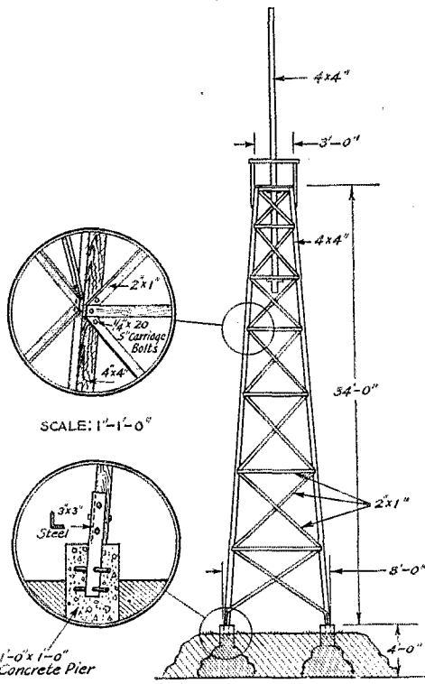
SCALE: 1" = 4'-0"
