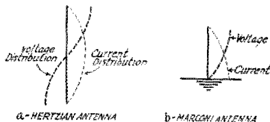
FIG 3 - ANTENNAS
