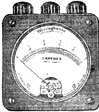
TYPE PX-3
