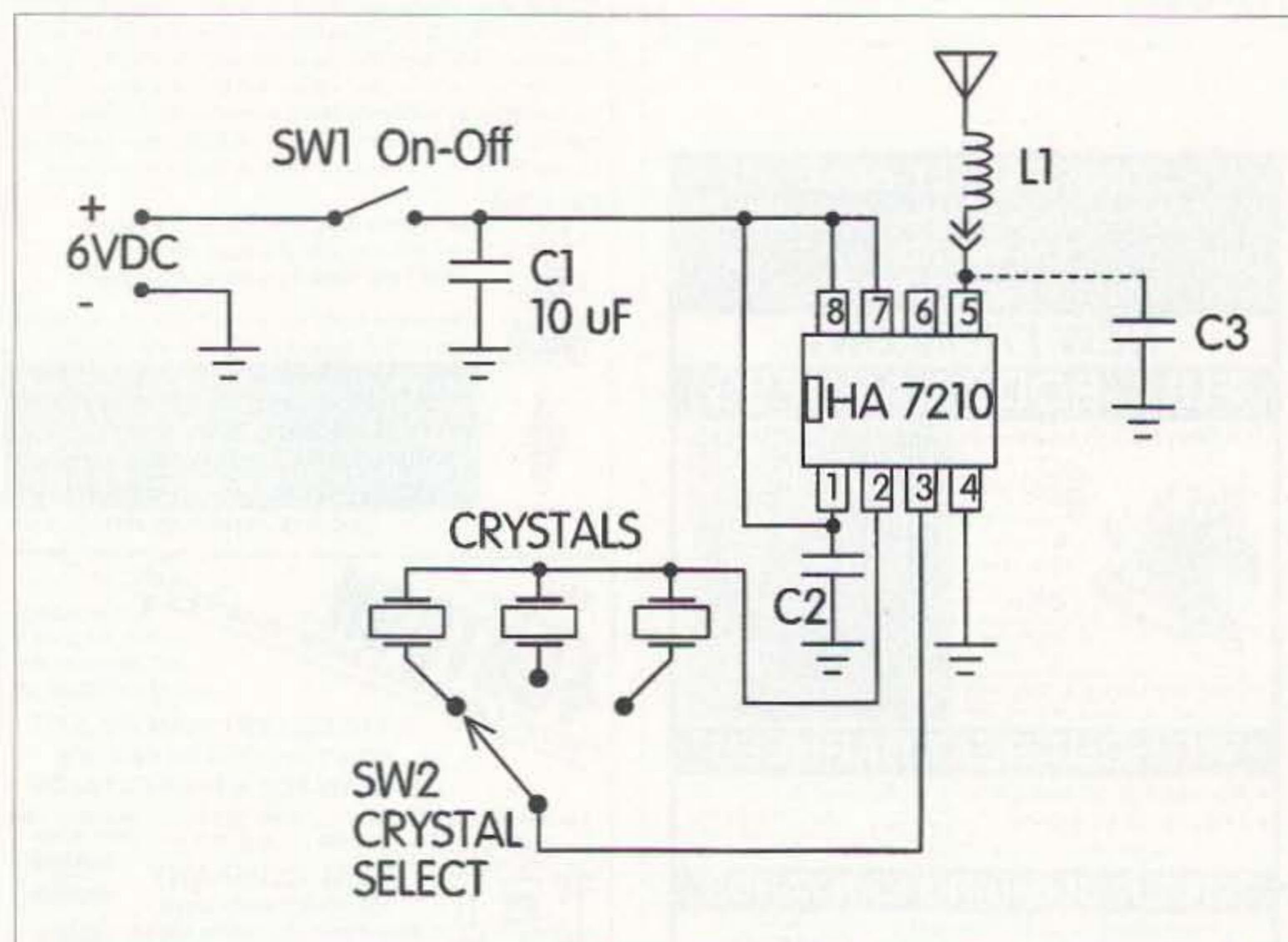
Fig. 1. The circuit.
