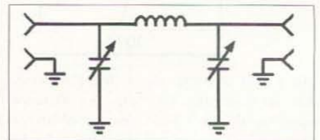
Fig. 2. Pi-match.
