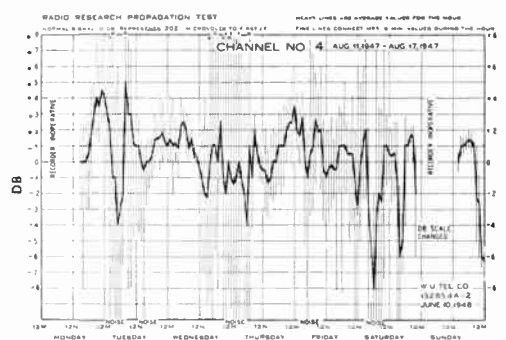
(d) Hourly fading data on 3.1 cm, August 11-17, 1947
