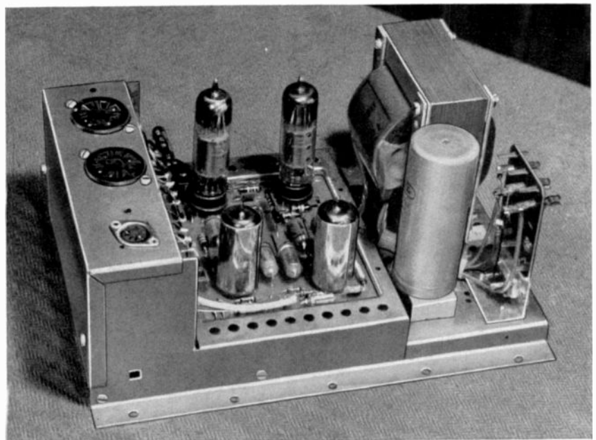
Bild 3 NF 1 bei abgenommener Haube
