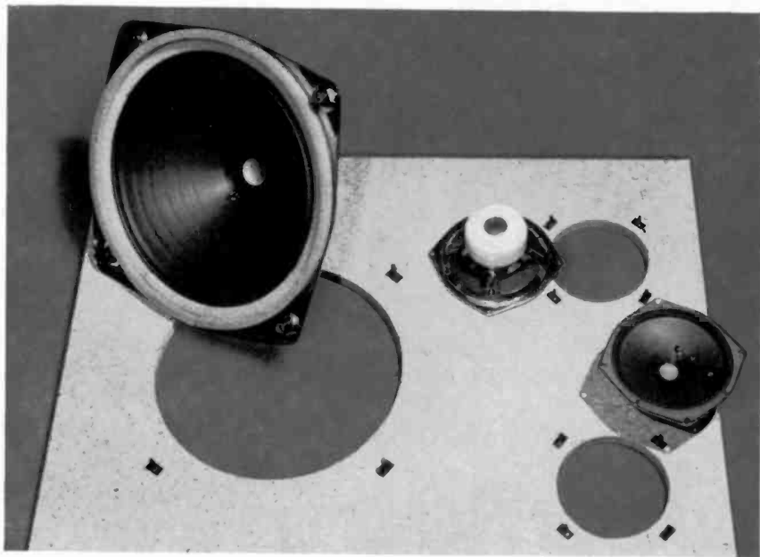
GRUNDIG Baflautsprecher 7003 (die Schaumstoffaufhängung der Membrane ist deutlich zu erkennen!) und zwei Hochtöner-Lautsprecher 7014, also eine Hälfte der Lautsprecherbestückung von LS 31, zusammen mit vorbereiteter Schallwand
