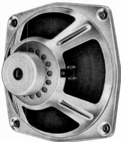
Typ 7003 Der berühmte GRUNDIG Baßlautsprecher 27 cm Ø. In Schaumstoff eingefasste Membrane
