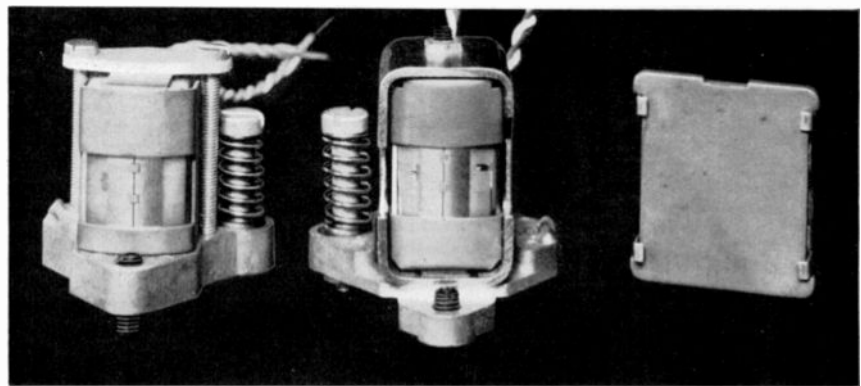
Bild 3 Viertelspur-Sprechkopf (lks.) und Viertelspur-Hörkopf. Rechts die Mu-Metall-Abschirmkloppel des Hörkopfes.
