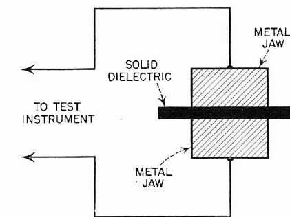
SIMPLE METAL-JAW TEST CAPACITOR FIG. 1
