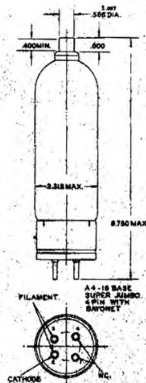
TYPE 8008XE
