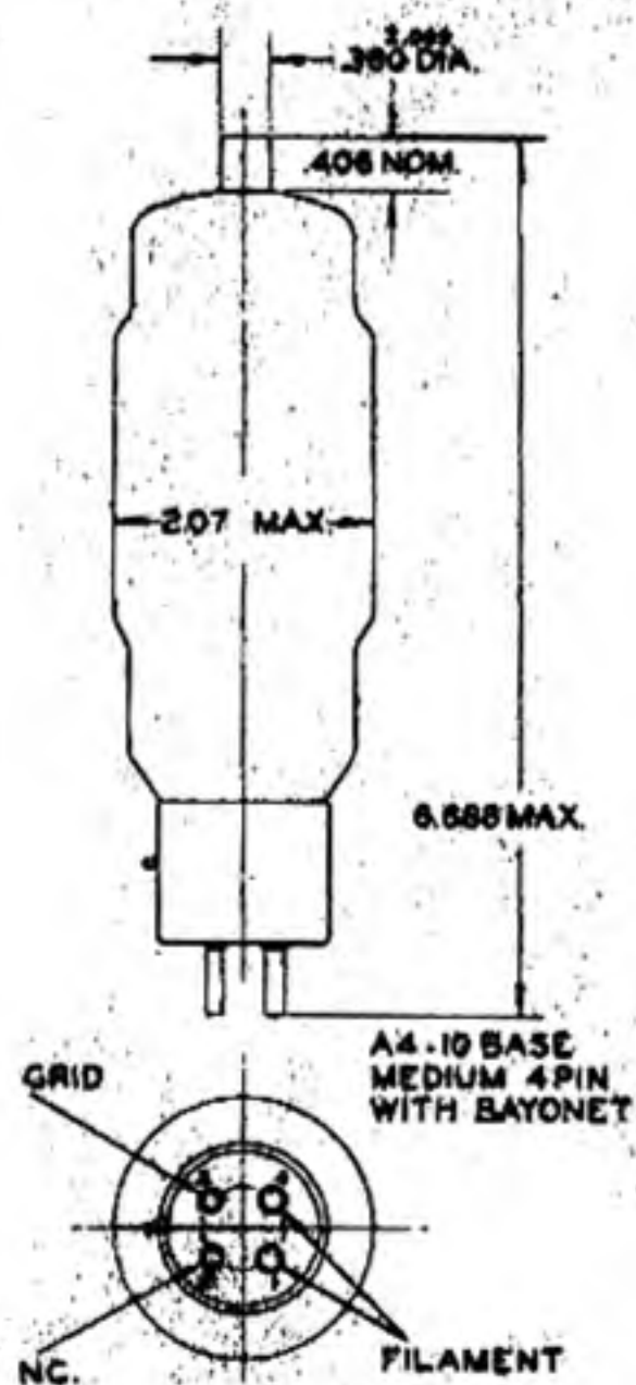
TYPE 830B
