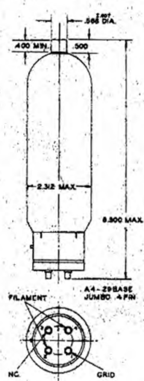
TYPE 805
