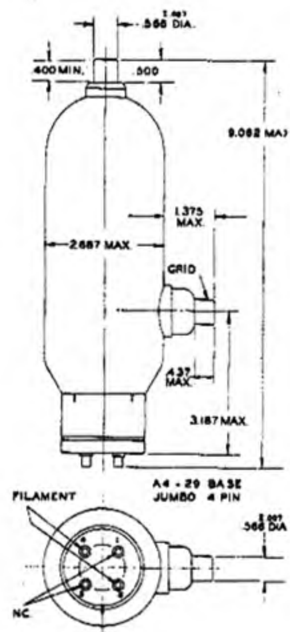
TYPE FV-20
