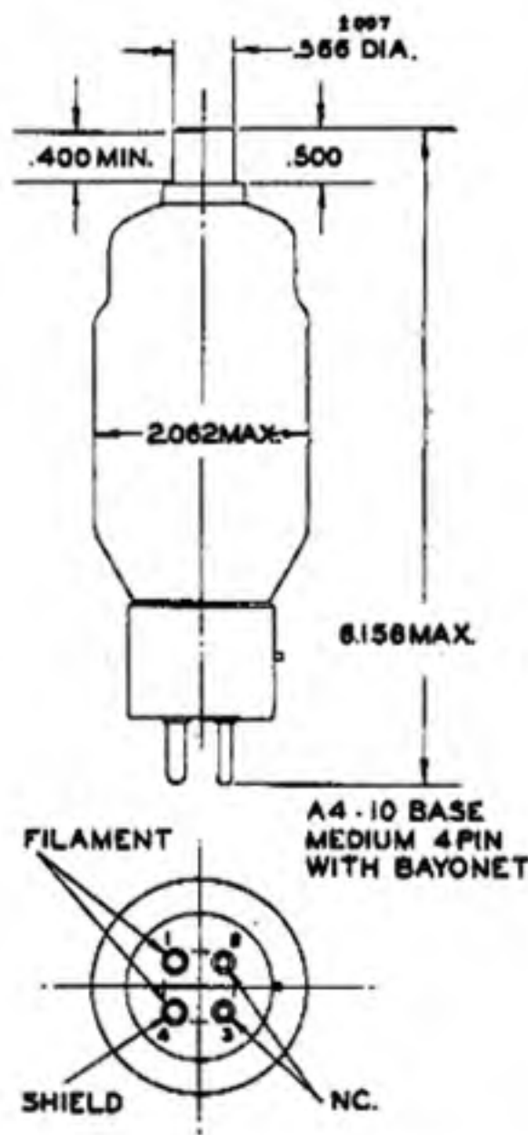
TYPE 3B28
