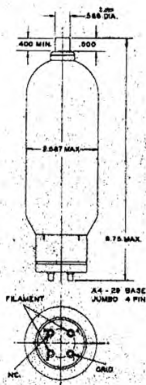
TYPE 311CH
