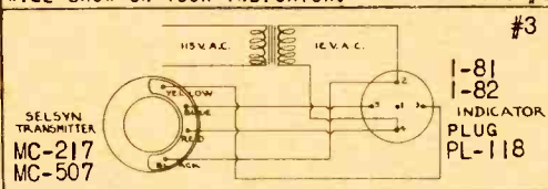
WIRING DIAGRAM FOR 115/90 VOLT SELSYN/SYNCHRO
