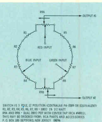
Fig. 5 Chroma Keyer matrix.
