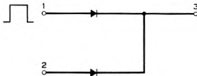
Fig. 1 — Diode or circuit.
