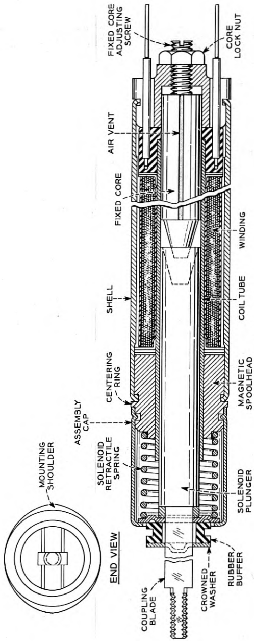
Fig. 33 — Solenoid.
