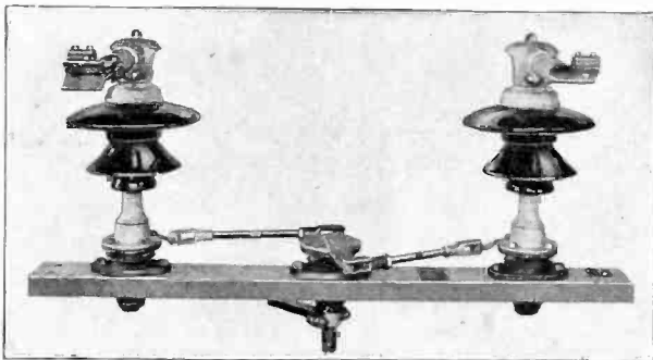
Unit Type PM-Form 2, 37 K.V., 600 Amperes
